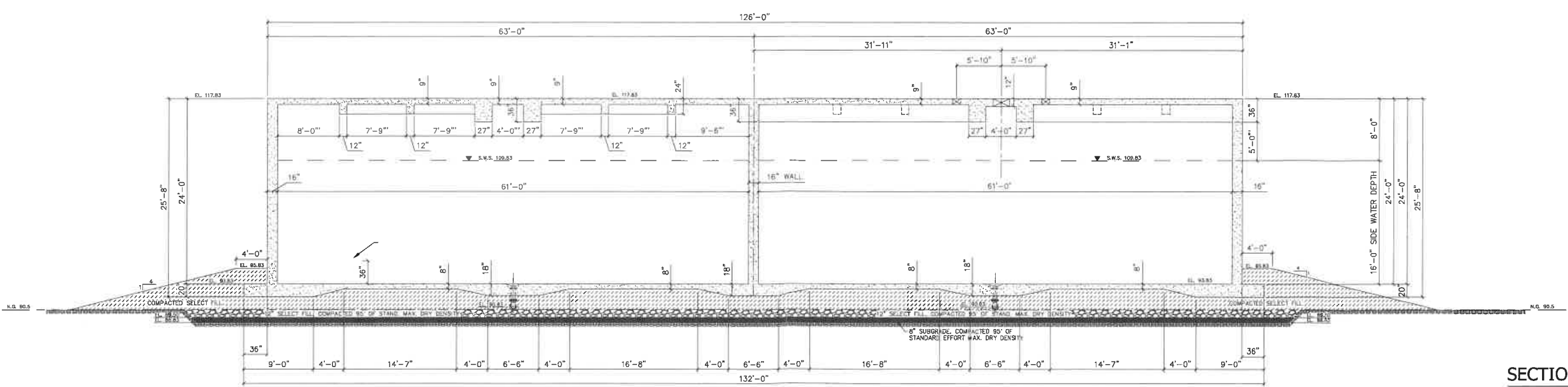
SECTION B SCALE: 1/8"=1'-0"
